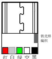
Micro usb母头焊接面
