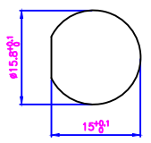
面板开孔尺寸
