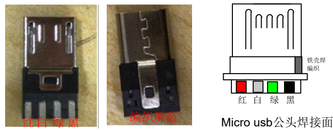
公头线束焊接实物图
